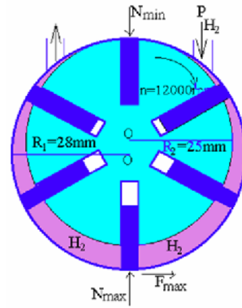
气动机示意图
