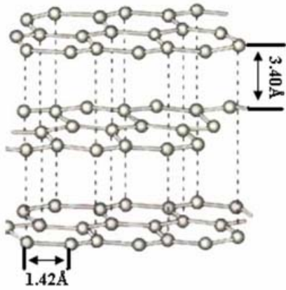
石墨的结构模型
