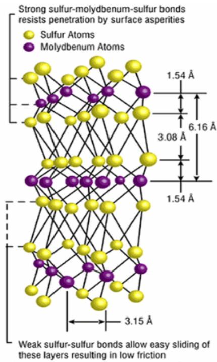
二硫化钼的结构模型
