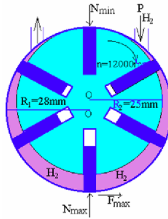
气动机示意图
